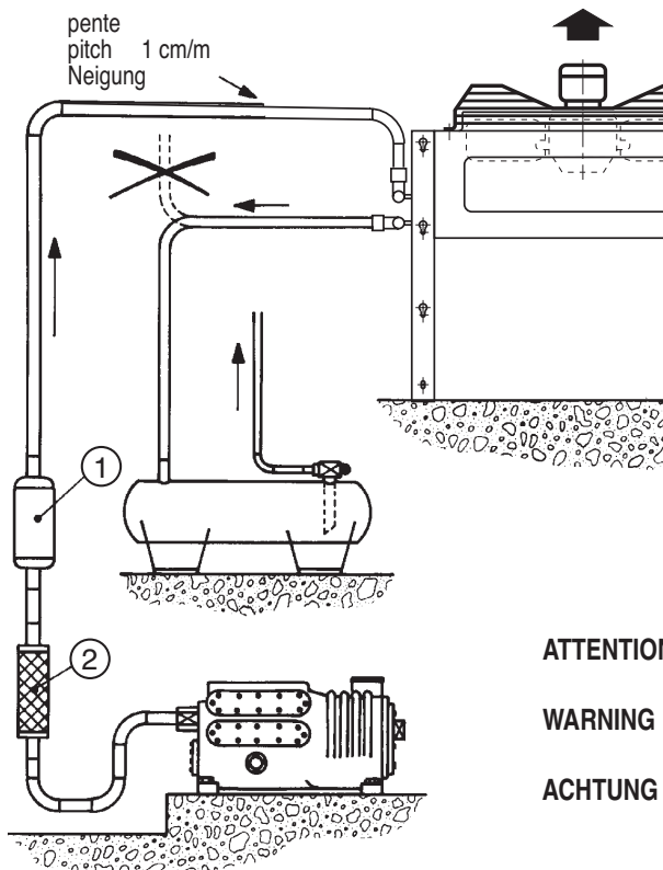
Schéma "type" d'installation - Typical piping - Montageschema
